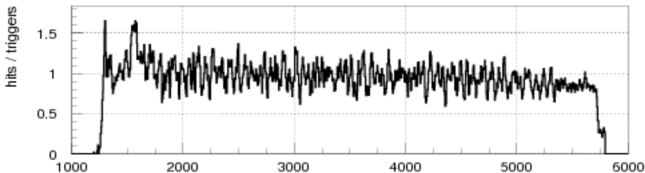
Fig. 11b spill time (ms)
