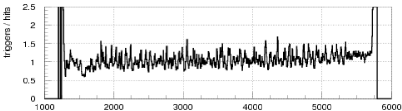
Fig. 11c spill time (ms)
