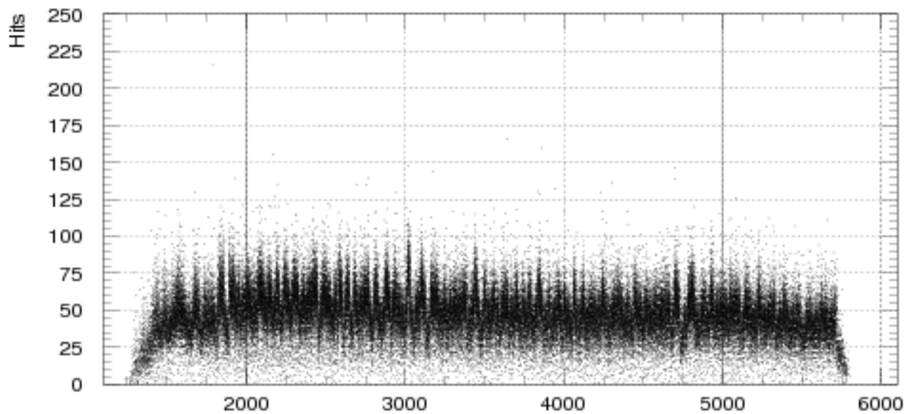
Fig. 6 Spill Time (ms)
