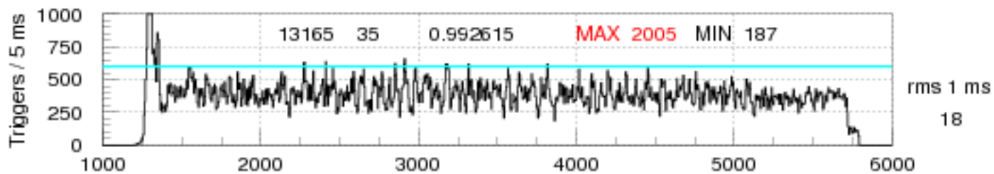
Fig. 1 spill (ms)
