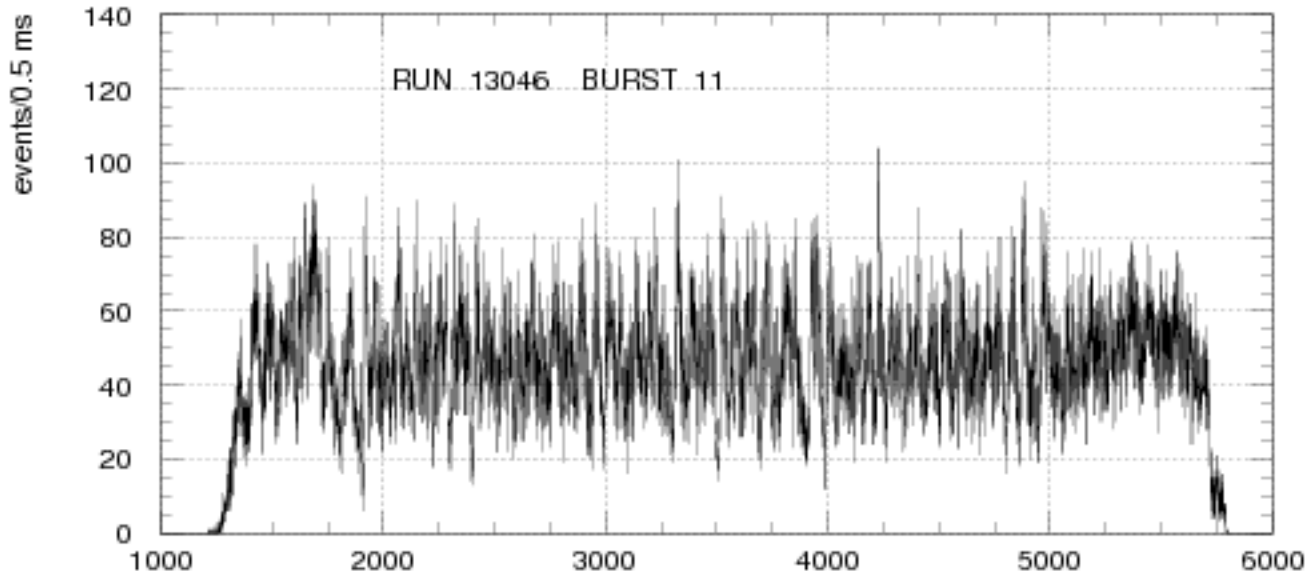
Fig. 1 Spill in 0.5 ms bins
